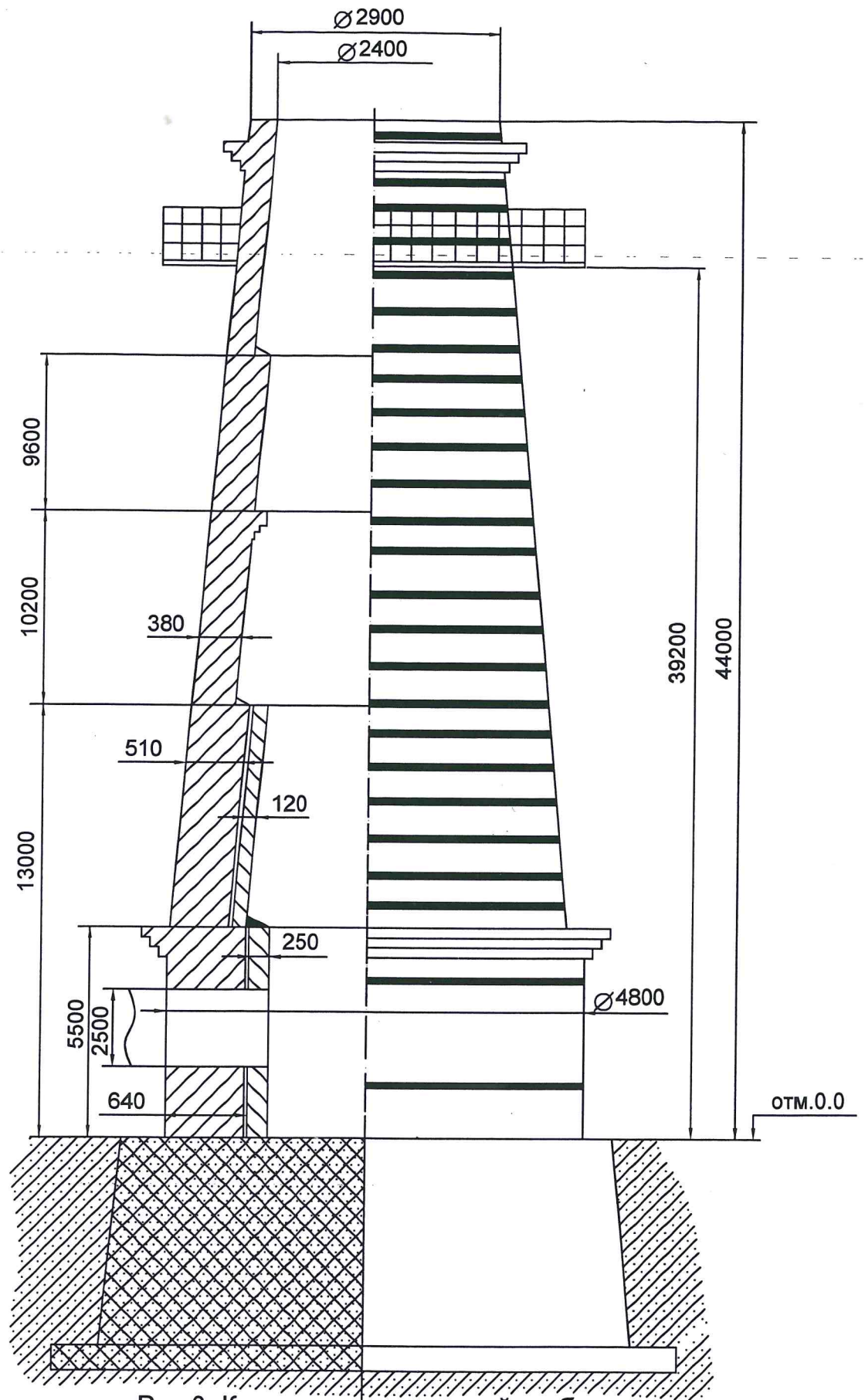
Рис. 3. Конструкция кирпичной трубы.
